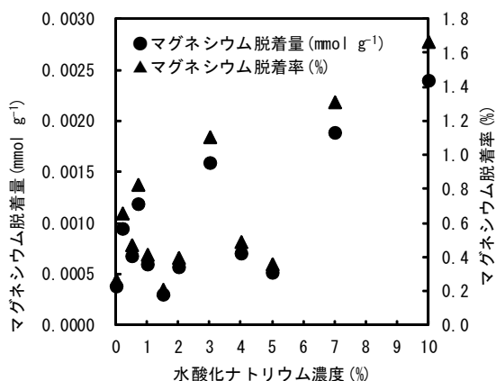
図3 水酸化ナトリウム溶液によるマグネシウムの脱着
