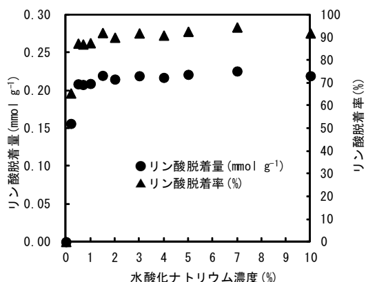
図1 水酸化ナトリウム溶液によるリンの脱着
