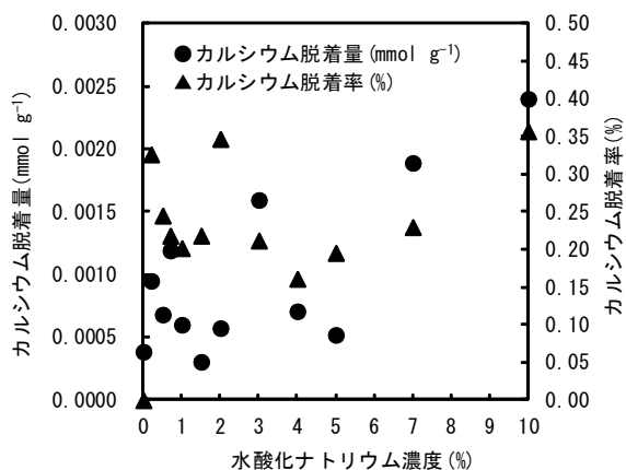
図6 水酸化ナトリウム溶液によるカルシウムの脱着
