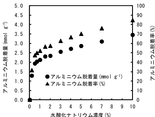
図4 水酸化ナトリウム溶液によるアルミニウムの脱着
