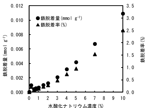
図5 水酸化ナトリウム溶液による鉄の脱着
