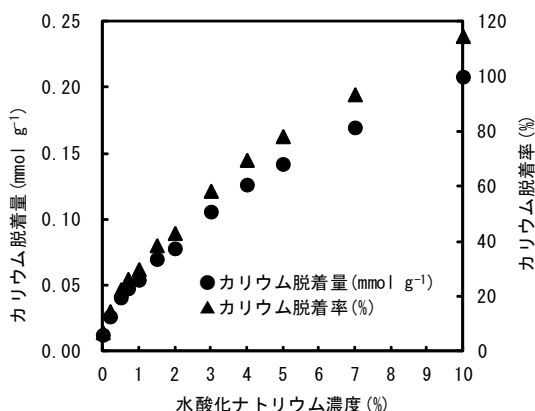
図2 水酸化ナトリウム溶液によるカリウムの脱着
